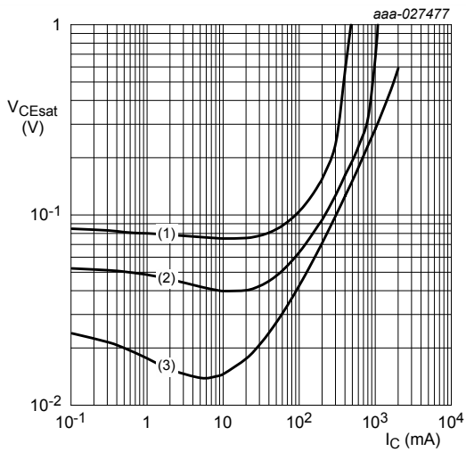
T_{amb} = 25\text{ }^\circ\text{C} (1) I_C/I_B = 50 (2) I_C/I_B = 20 (3) I_C/I_B = 5
